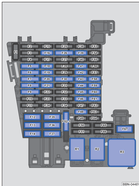
图 157 仪表板中：保险丝分配
