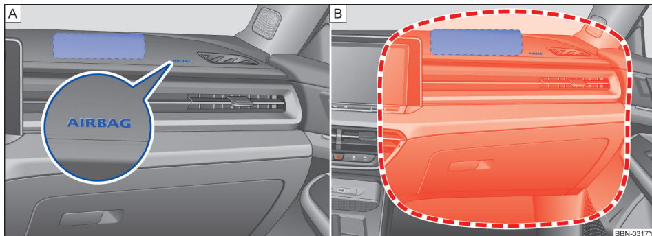
图 34 副驾驶员前部安全气囊的安装位置和膨胀范围
