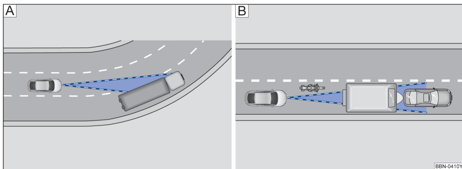
图 109 [A]. 处在弯道里的汽车；[B]. 前方行驶的摩托车处在雷达传感器探测范围外
