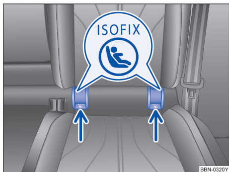
图 38 汽车座椅上的儿童座椅下部固定点标记。
