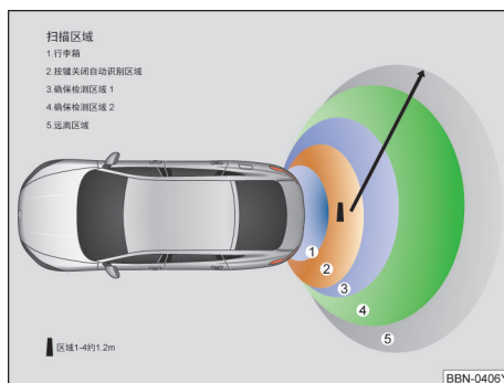
图 60 感应式行李厢盖开启和关闭钥匙有效识别区域
