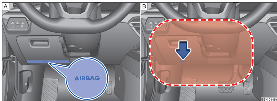
图 37 驾驶员侧：膝部安全气囊安装位置及作用范围
