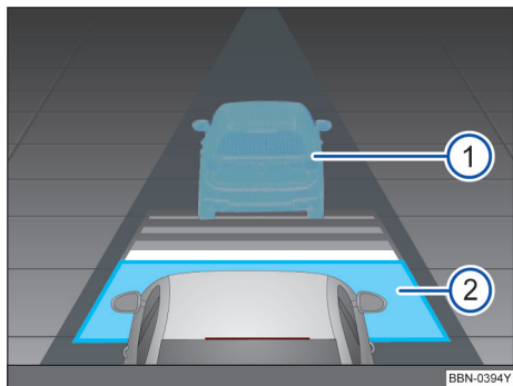
图 104 组合仪表显示屏：已暂时关闭自适应巡航系统（ACC）控制功能，已探测到的前方车辆，设定的距离间隔
