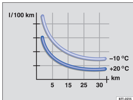
图 99 两种不同环境温度时的百公里油耗
