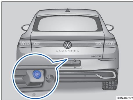
图 129 车辆行李厢盖内：倒车摄像头的安装位置
