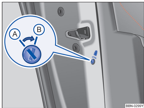
图 51 在左后车门中：儿童安全锁 (A) 已关闭、(B) 已接通
