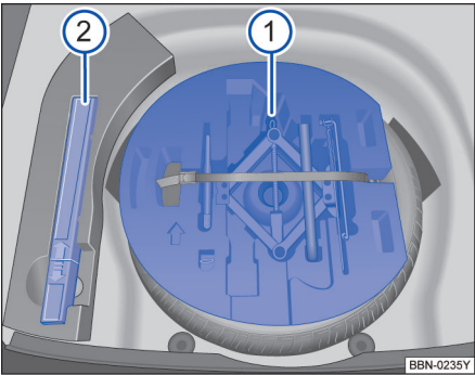
图 150 行李厢垫下的备用轮胎及随车工具
