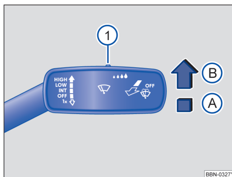
图 88 车窗玻璃刮水器操作杆：调节雨量传感器
