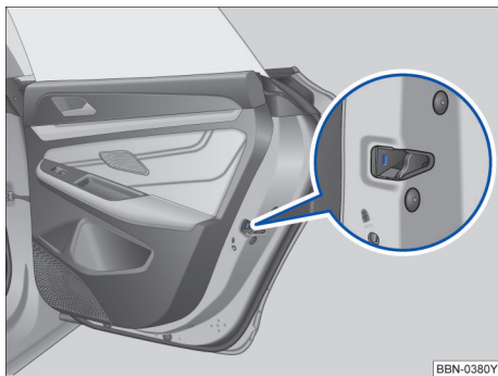
图 54 右侧后车门端面处的应急上锁装置
